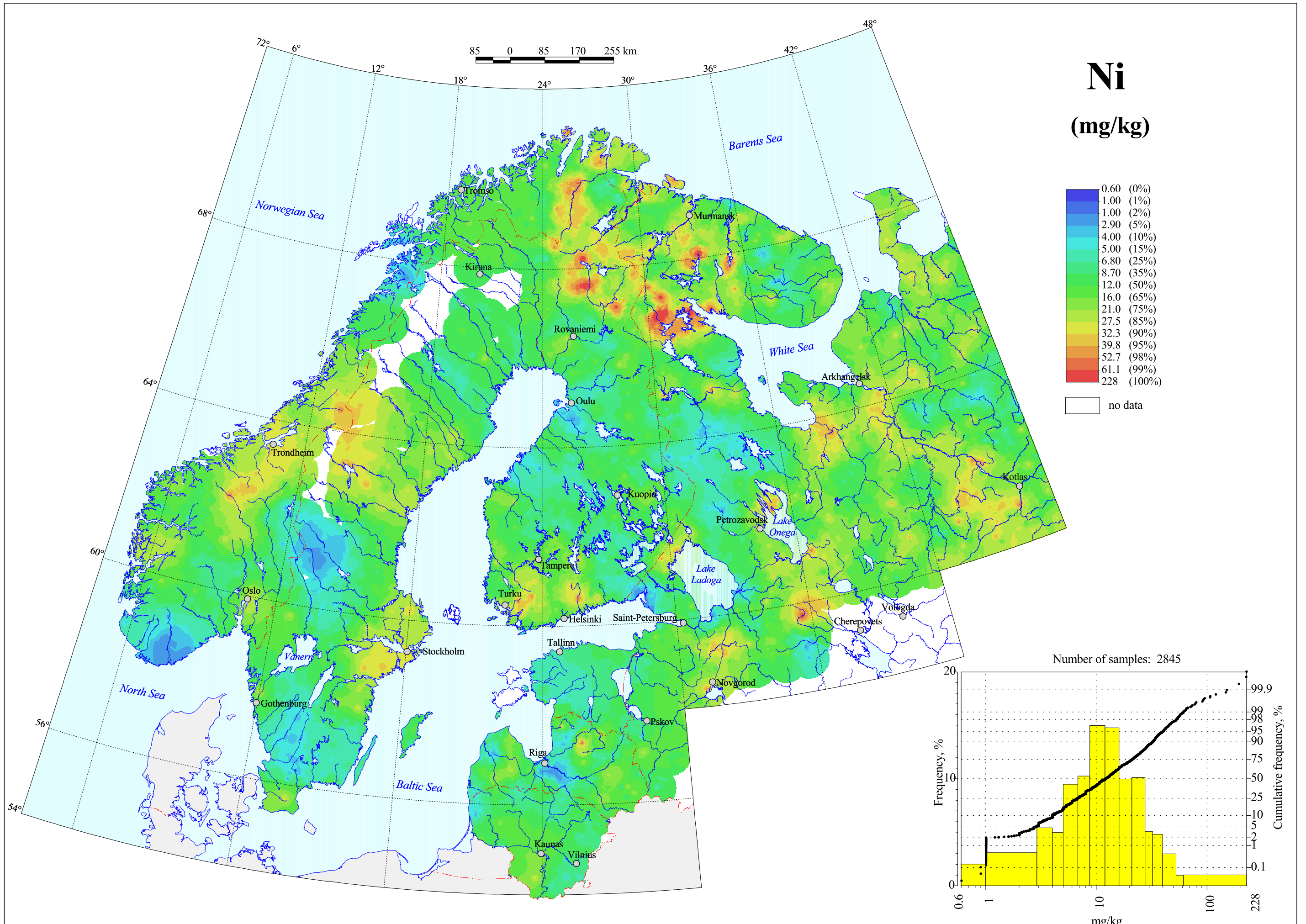
Nickel in C-horizon, Grain Size <2 mm, Aqua regia Extraction
